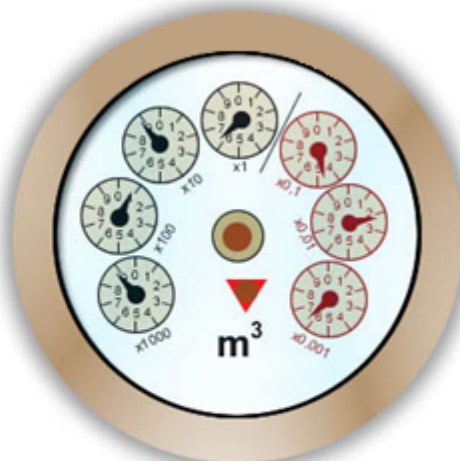
2) CONTATORE A LANCETTE
