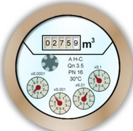
1) CONTATORE A LETTURA DIRETTA
