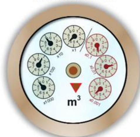
2) CONTATORE A LANCETTE
